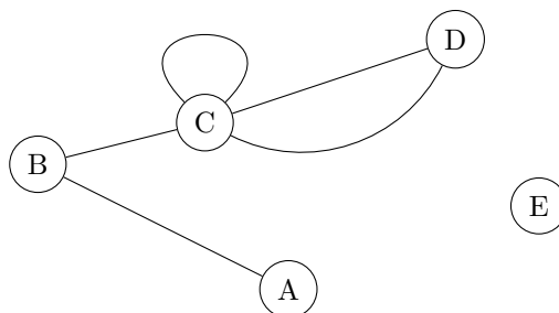
Figur 2: Illustration af begreberne i definition 1.1. A og B er et eksempel på to naboknuder. C har en løkke. E er en isoleret knude, idet denne knude ingen kanter har. Valensen af A er 1, for B er den 2. Valensen af C og D er henholdsvis 5 og 2.
